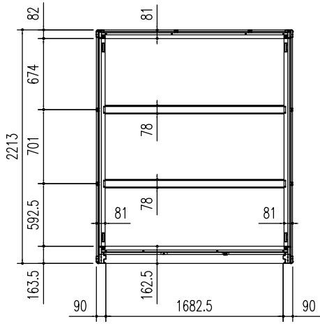
床伏図 (S = 1/50)
