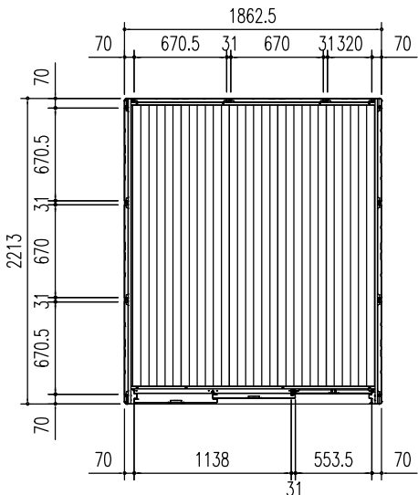
平面図 (S = 1/50)
