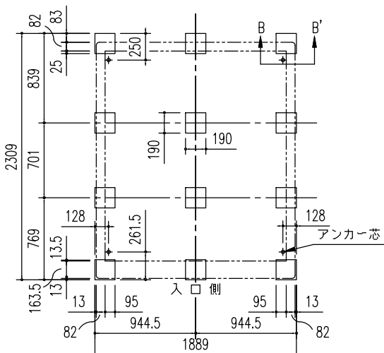
ブロック基礎図 (S = 1/50) (内アンカー用) ※内アンカーセット(オプション) 別途必要
