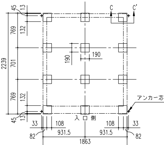
ブロック基礎図 (S = 1/50) (外アンカー用)
