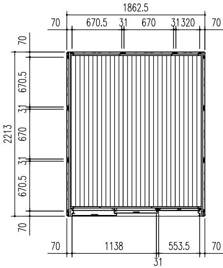
平面図 (S = 1/50)
