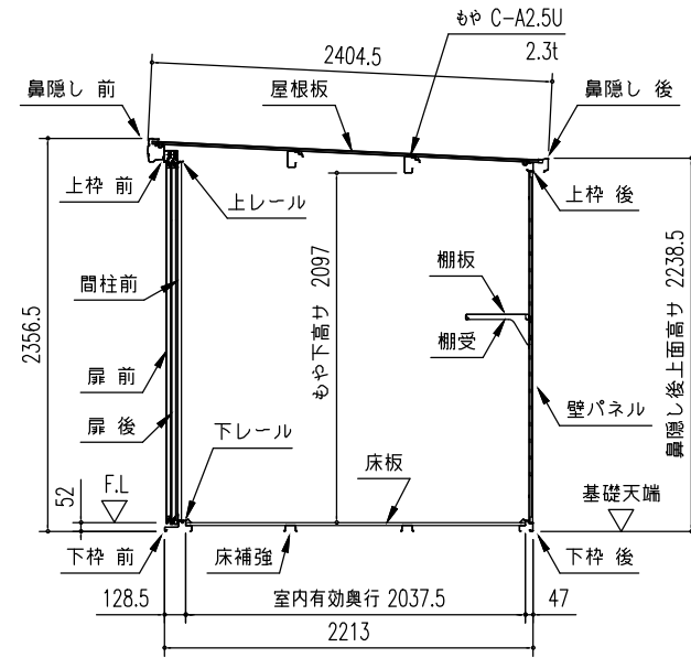
矩計図 (S = 1/50)
