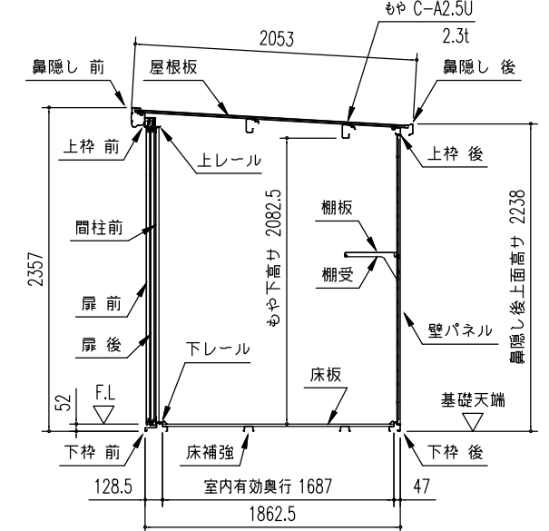
矩計図 (S=1/50)
