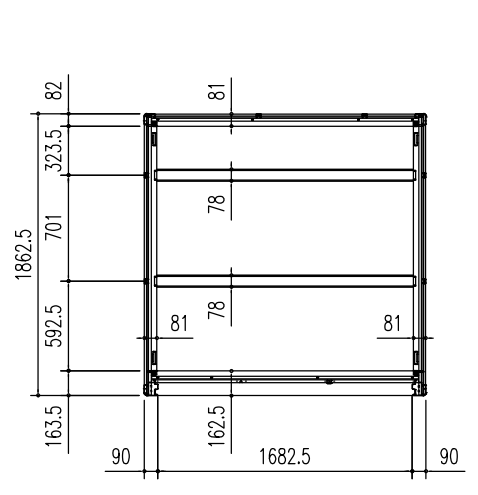
床伏図 (S=1/50)
