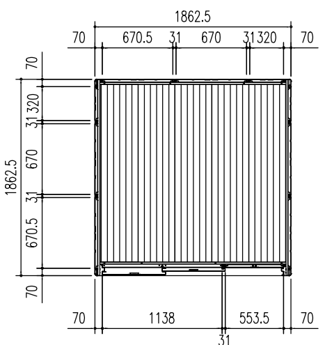
平面図 (S=1/50)
