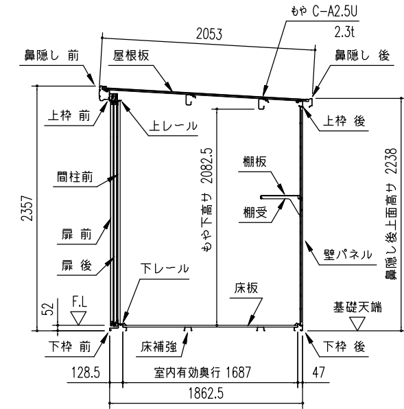
矩計図 (S=1/50)
