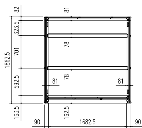
床伏図 (S=1/50)
