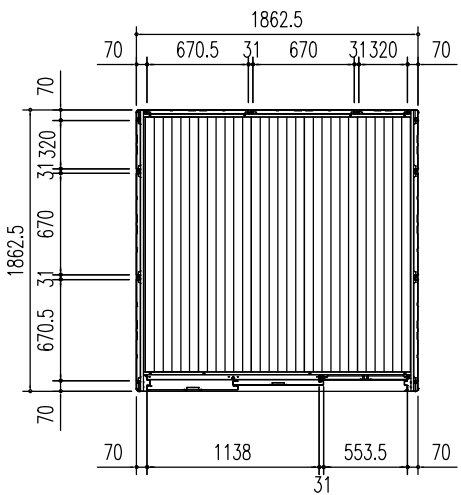
平面図 (S=1/50)
