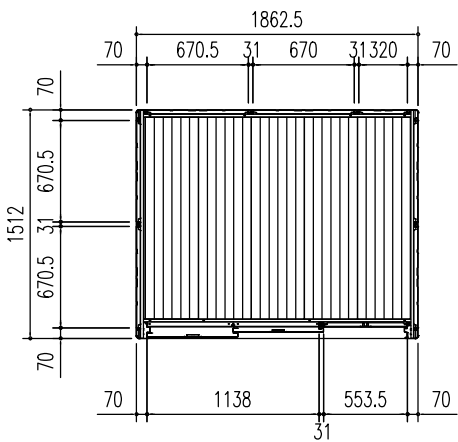
平面図 (S=1/50)
