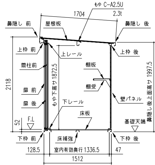
矩計図 (S=1/50)
