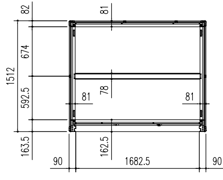
床 伏 図 (S=1/50)
