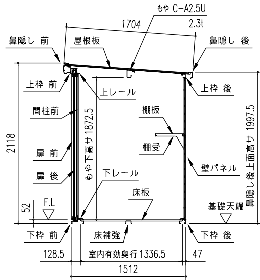
矩計図 (S=1/50)
