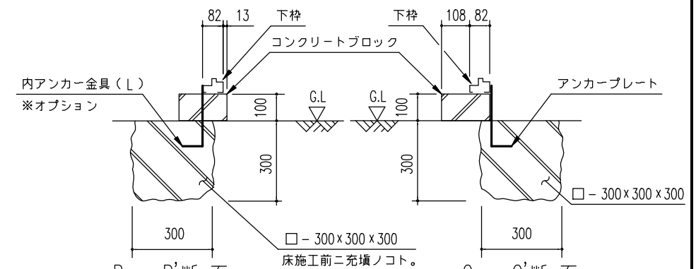
(内アンカー用)
