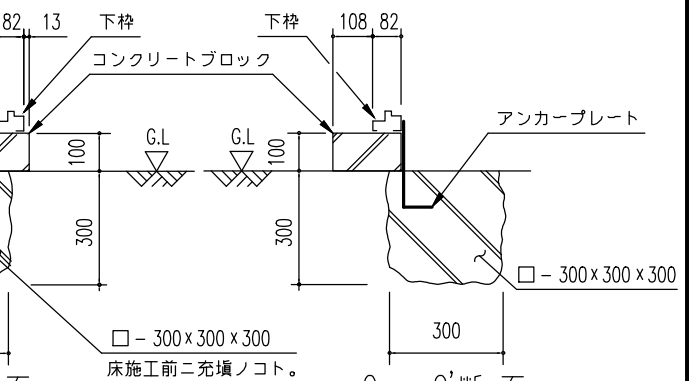
(外アンカー用)
