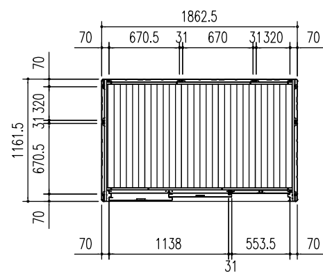
平面图 (S = 1/50)
