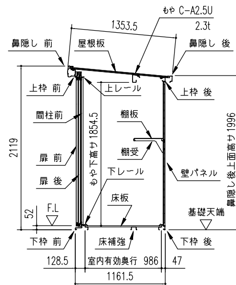
矩 計 図 (S = 1/50)
