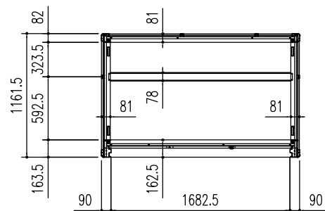
床 伏 図 (S = 1/50)
