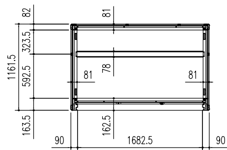
床伏図 (S=1/50)
