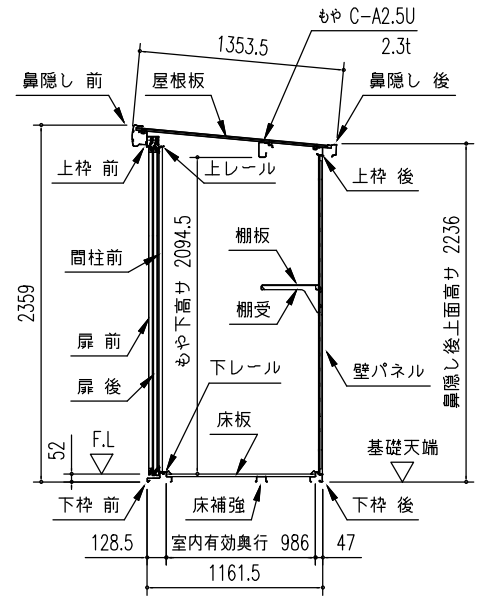
矩計図 (S=1/50)
