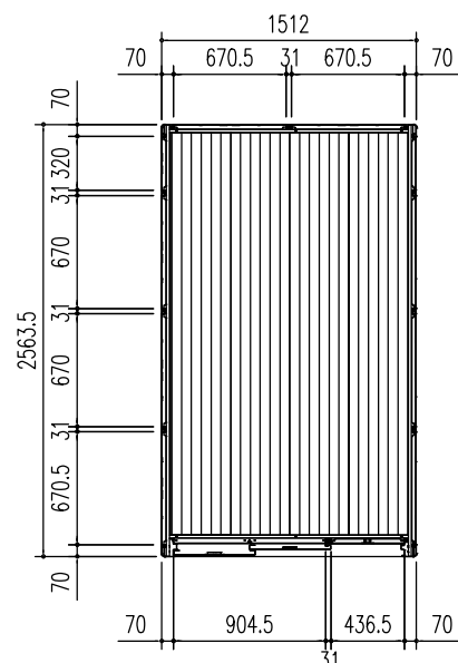
平面図 (S=1/50)
