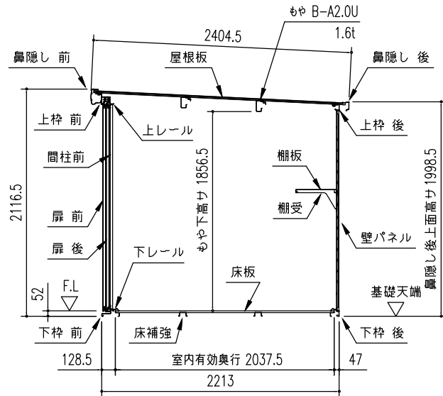
短計図 (S=1/50)
