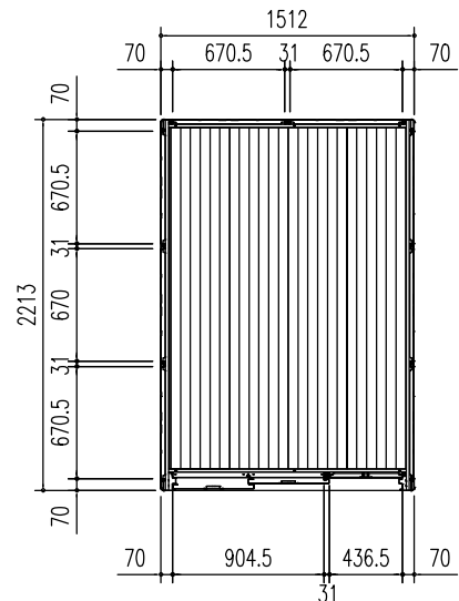
平面図 (S=1/50)
