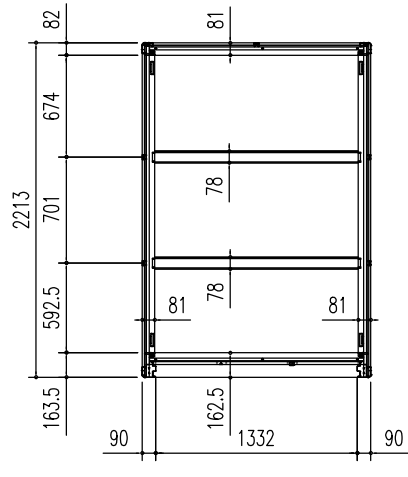
床伏図 (S=1/50)
