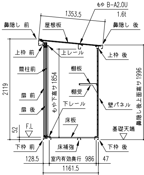
短計図 (S=1/50)
