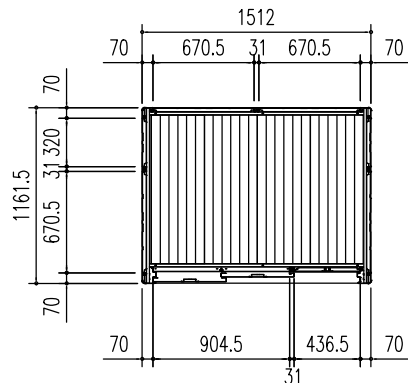
平面図 (S=1/50)
