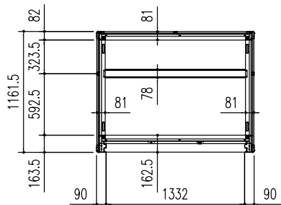
床伏図 (S=1/50)
