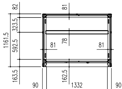
床伏図 (S=1/50)
