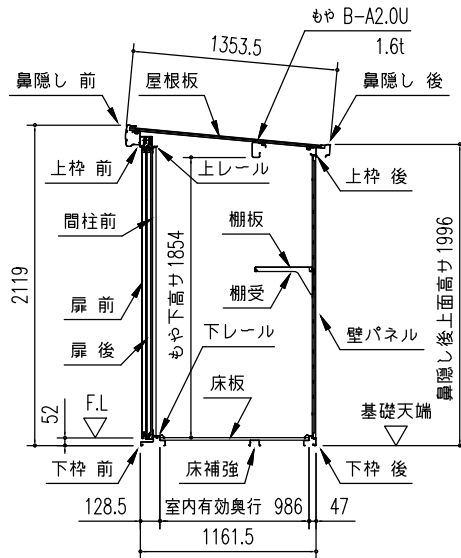
短計図 (S=1/50)
