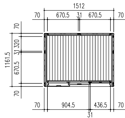
平面図 (S=1/50)
