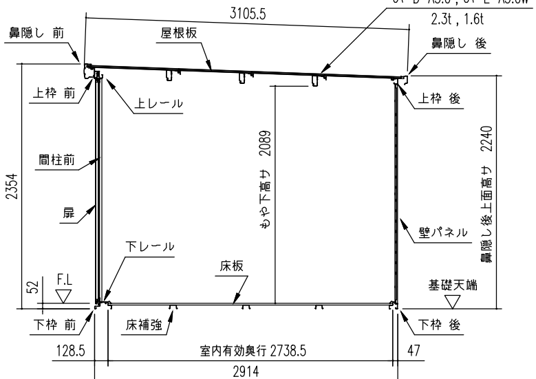
一般型矩計図 (S = 1/50)
