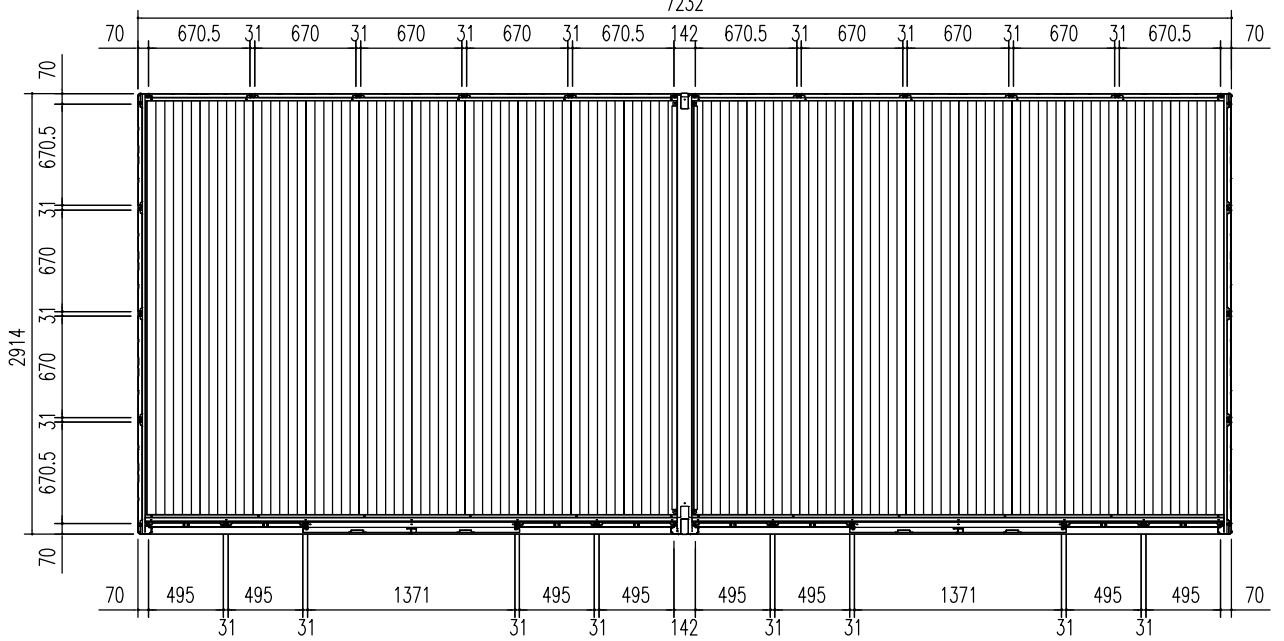
平面図 (S = 1/50)
