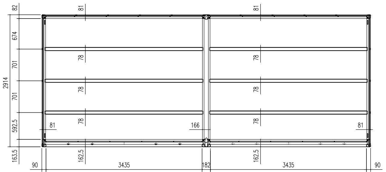
床伏図 (S = 1/50)
