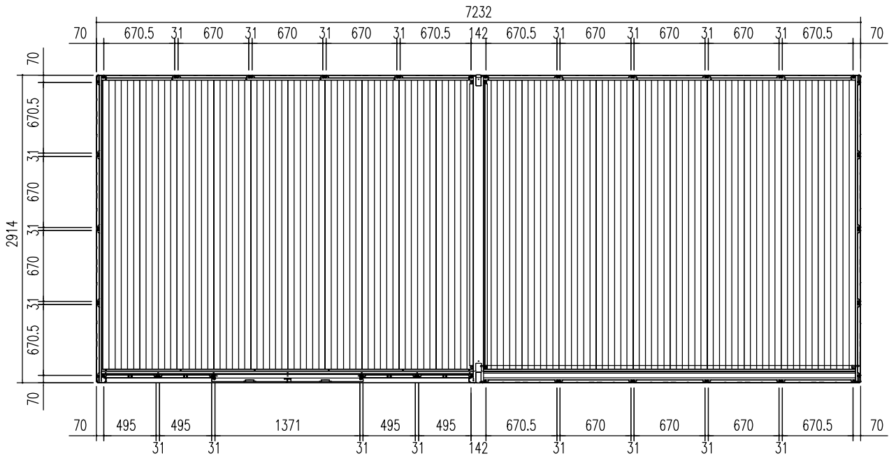
平面図 (S = 1/50)
