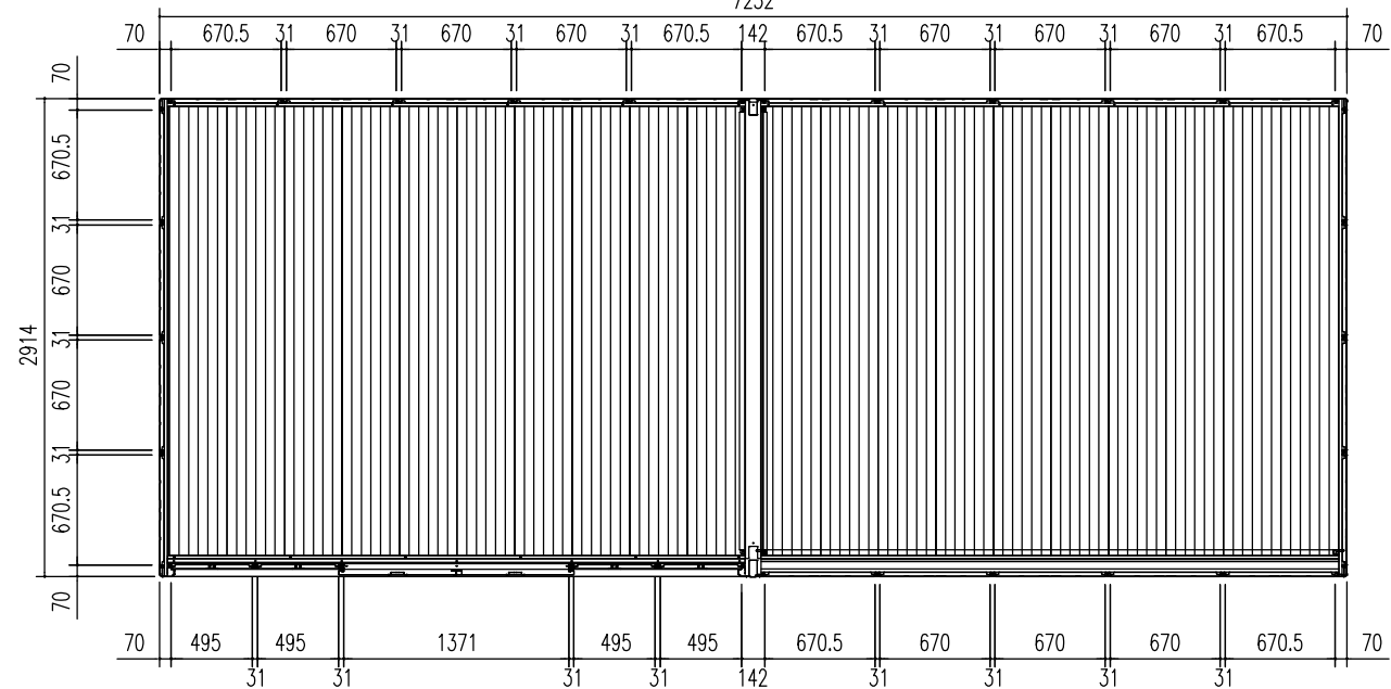
平面図 (S=1/50)
