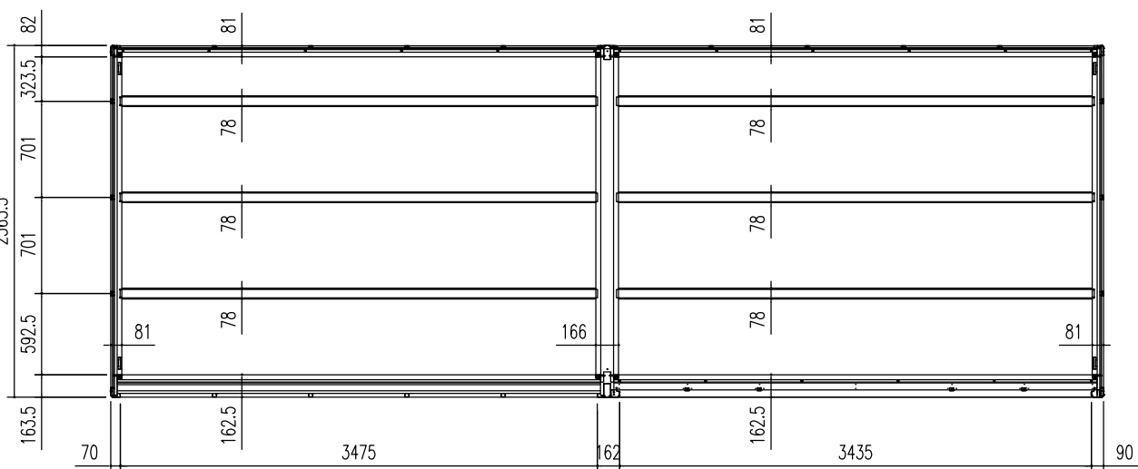
床 伏 図 (S = 1/50)
