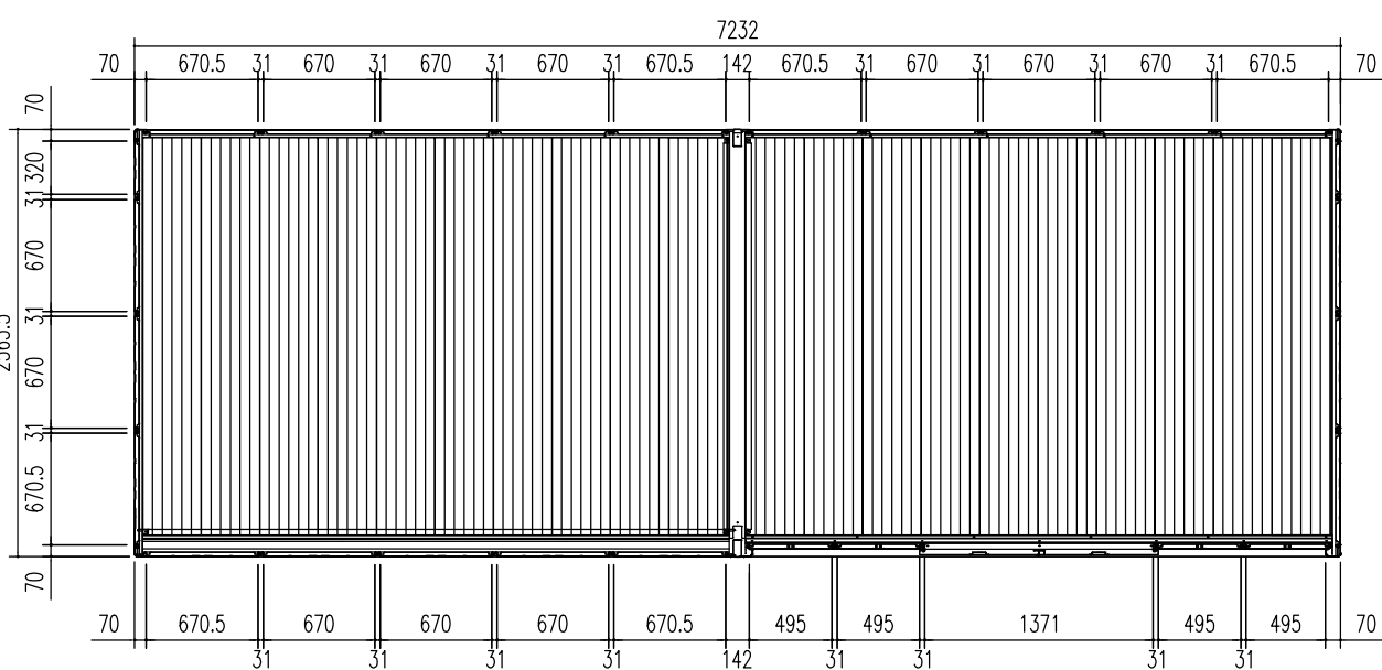
平面図 (S = 1/50)
