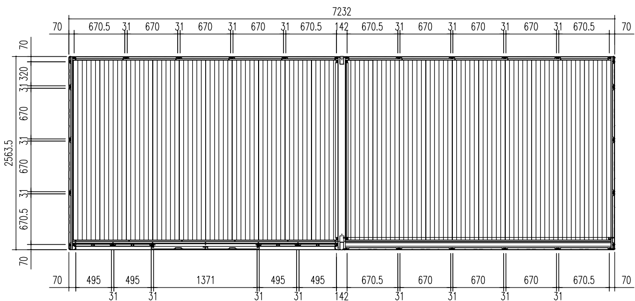
平面図 (S = 1/50)
