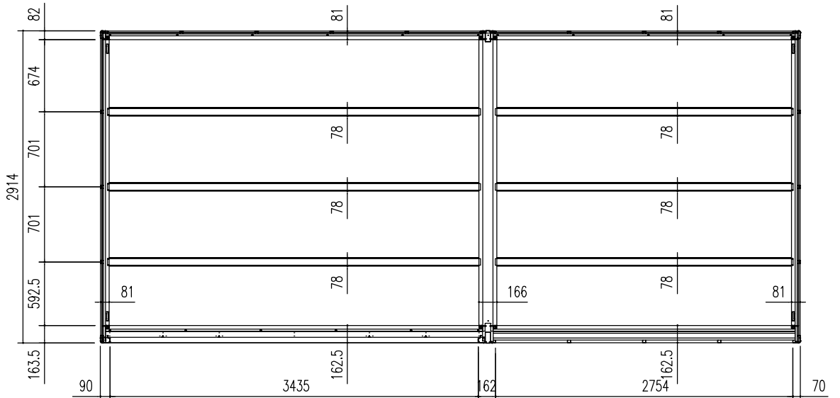
床伏図 (S = 1/50)
