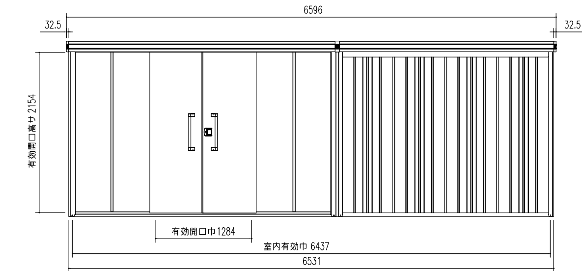
正面立面図 (S = 1/50)
