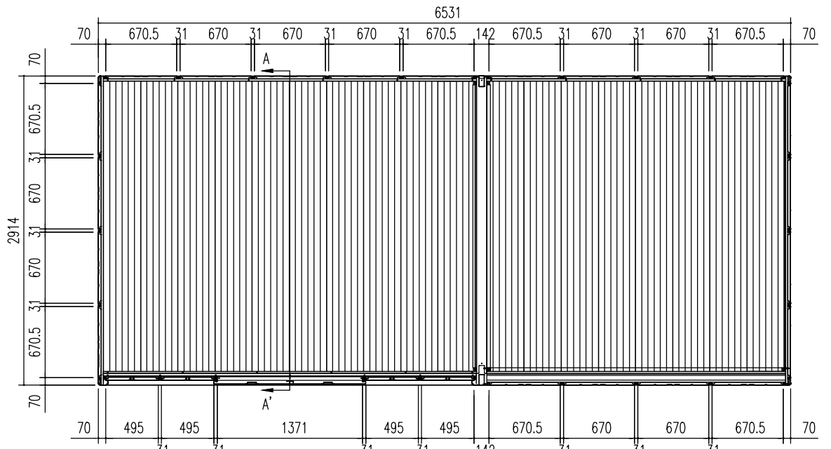
平面図 (S = 1/50)
