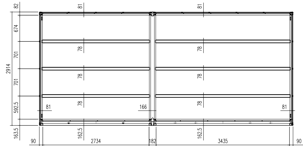
床伏図 (S = 1/50)
