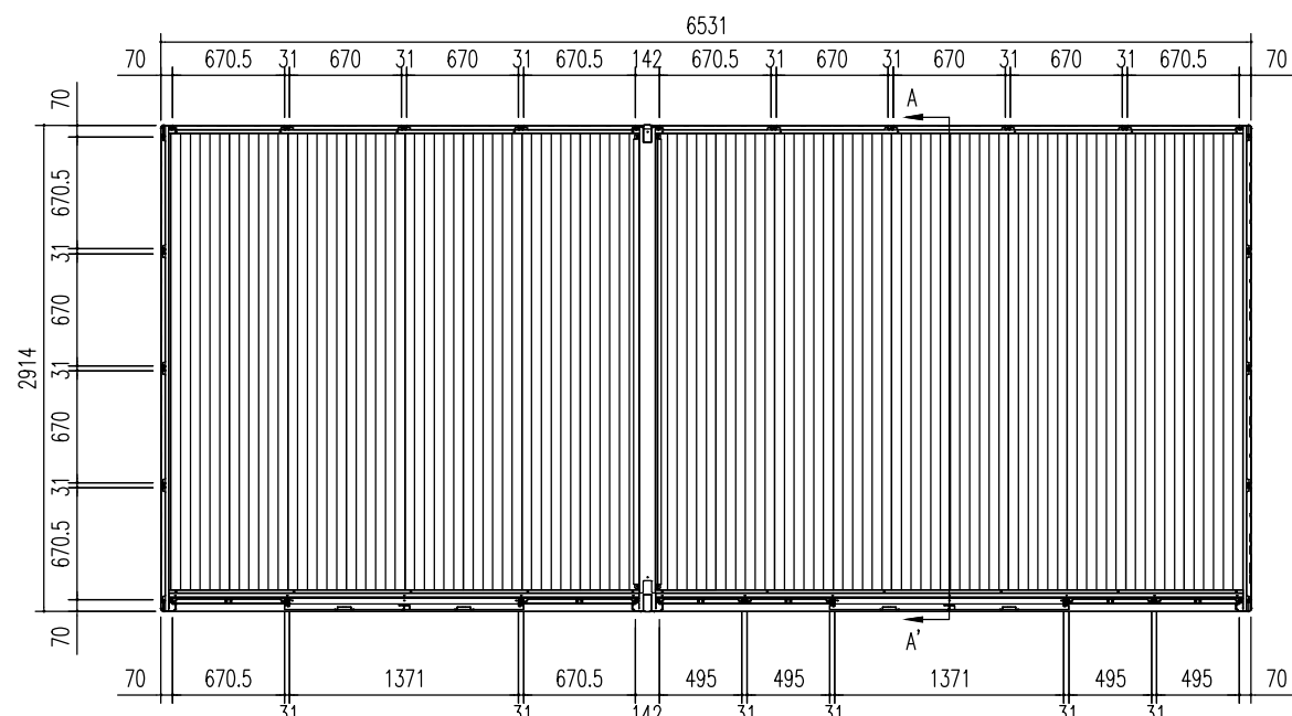
平面図 (s=1/50)
