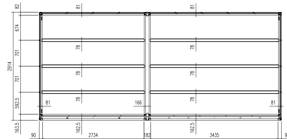
床伏図 (s=1/50)
