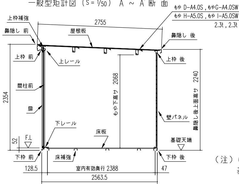
積雪型矩計図 (S = 1/50) A ~ A' 断面
