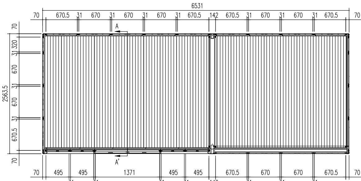
平面図 (S = 1/50)
