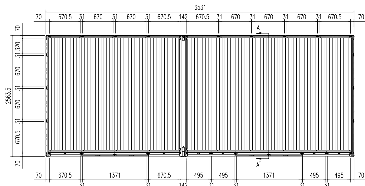
平面图 (S = 1/50)
