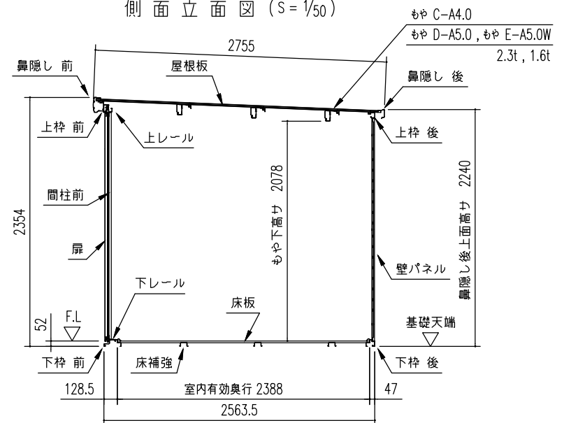
一般型矩計図 ( S = 1/50 ) A \sim A' 断面
