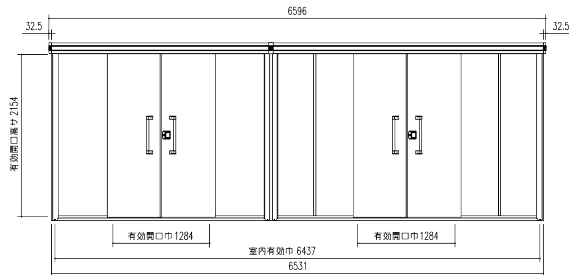
正面立面图 (S = 1/50)
