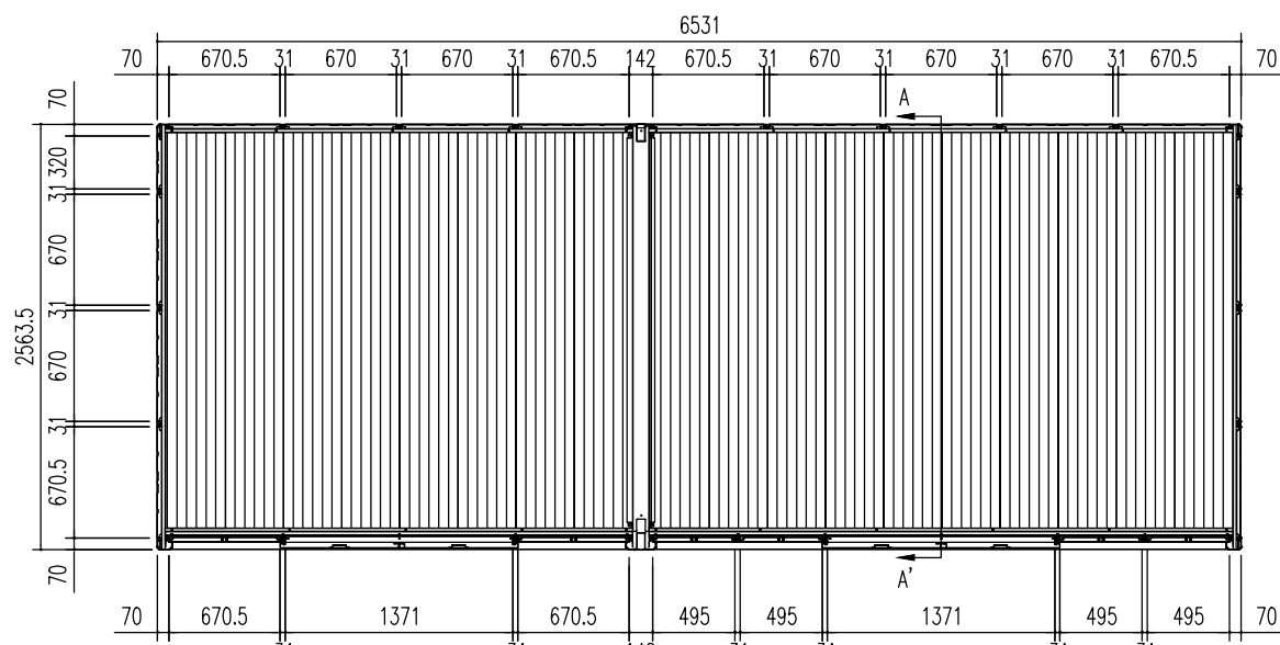
平面図 (s=1/50)
