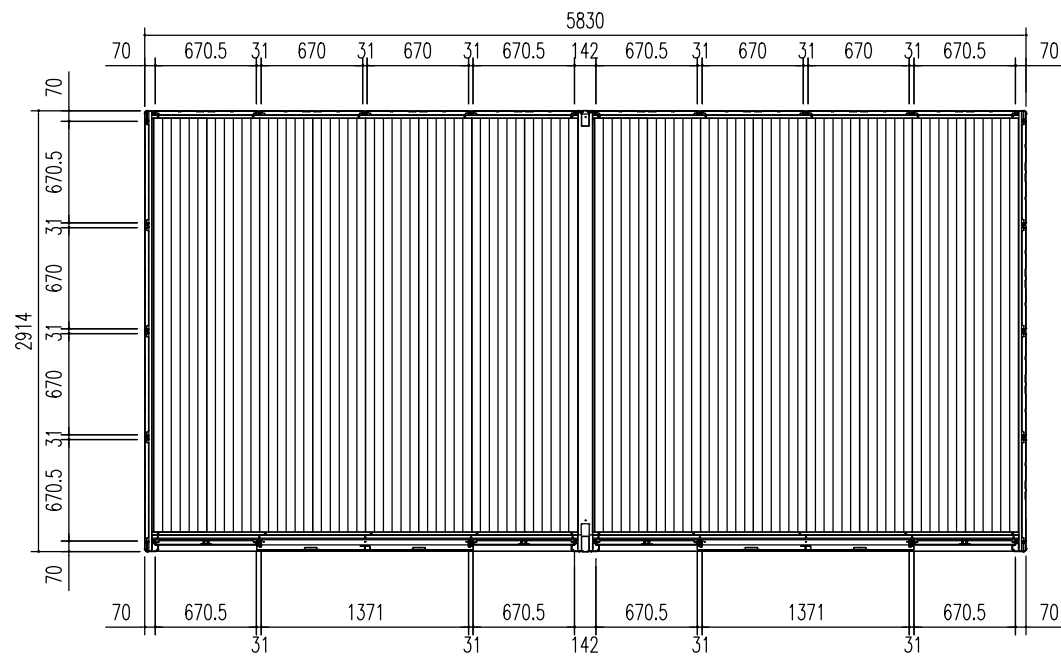
平面図 (S=1/50)
