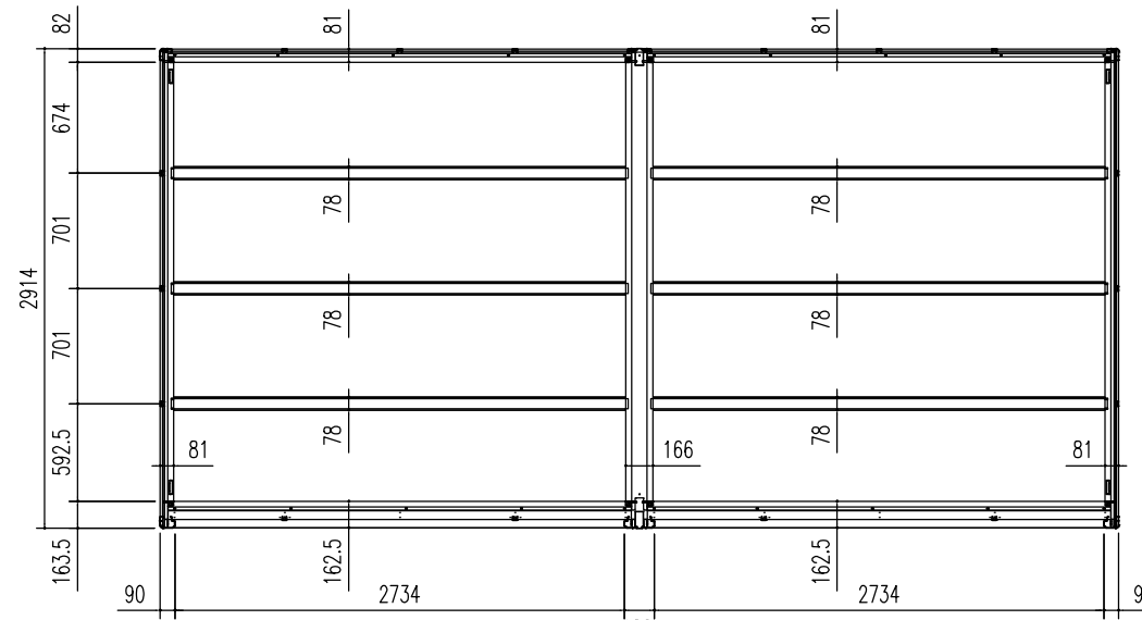
床伏図 (S=1/50)
