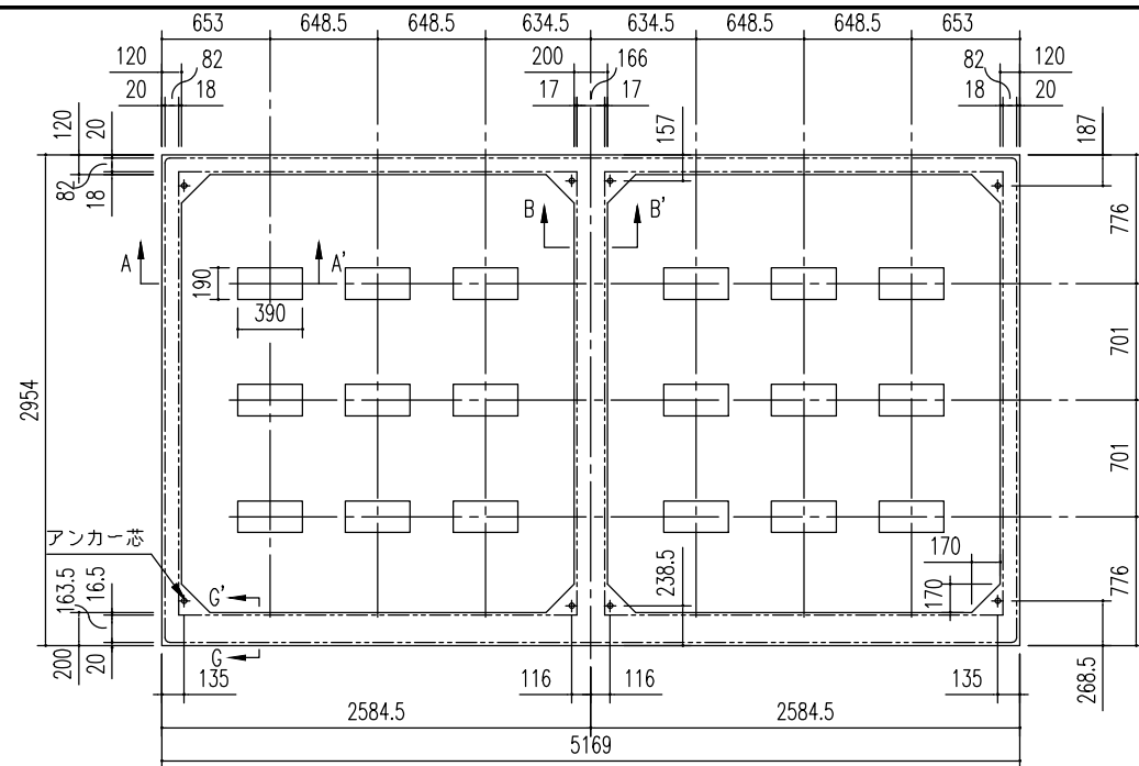
入口側 布基礎伏図 (S=1/50) ※内アンカーセット (オプション) 別途必要
