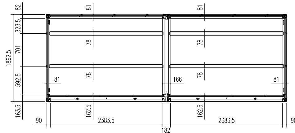
床伏図 (S = 1/50)
