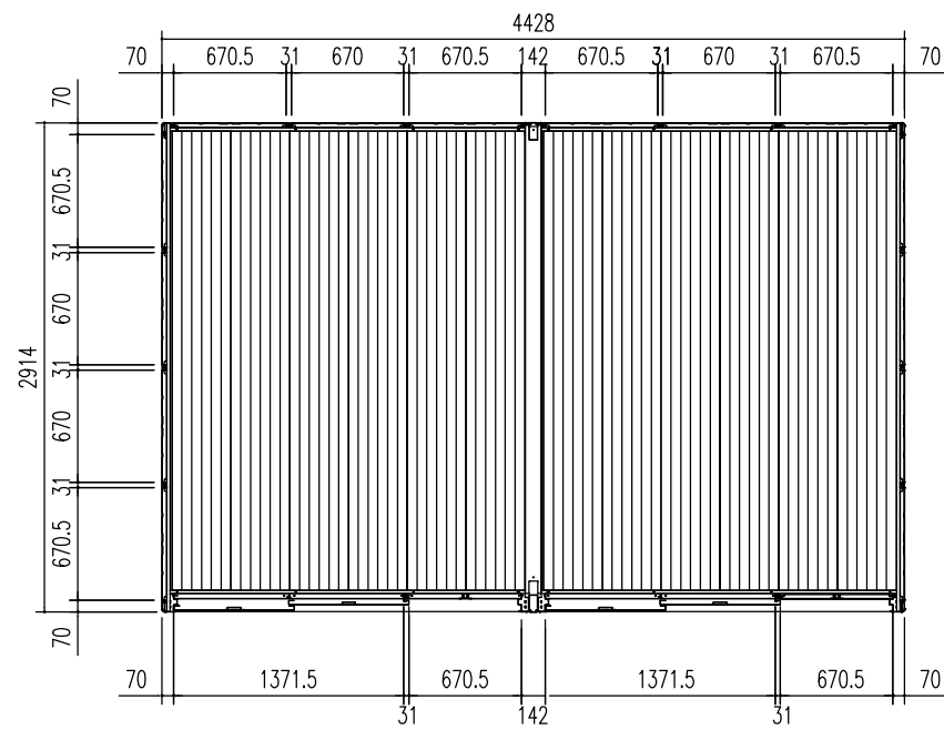
平面図 (S = 1/50)
