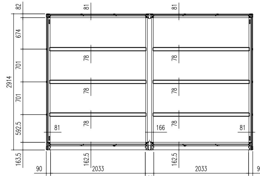
床伏図 (S = 1/50)
