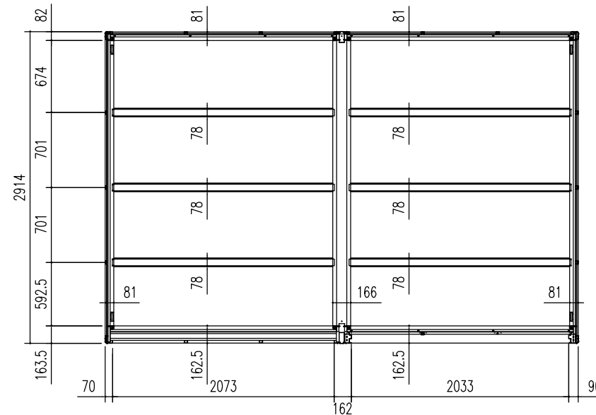
床伏図 (S=1/50)
