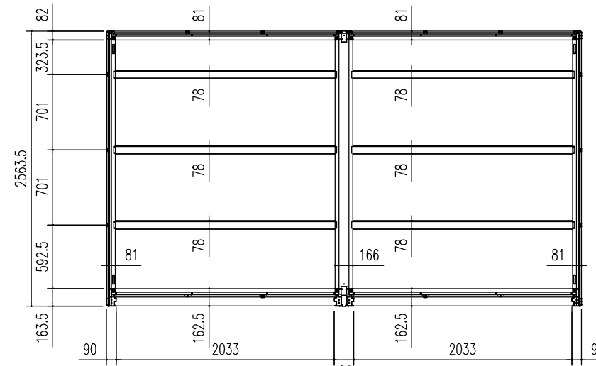
床伏図 (S = 1/50)
