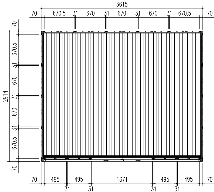
平 面 図 (S = 1/50)
