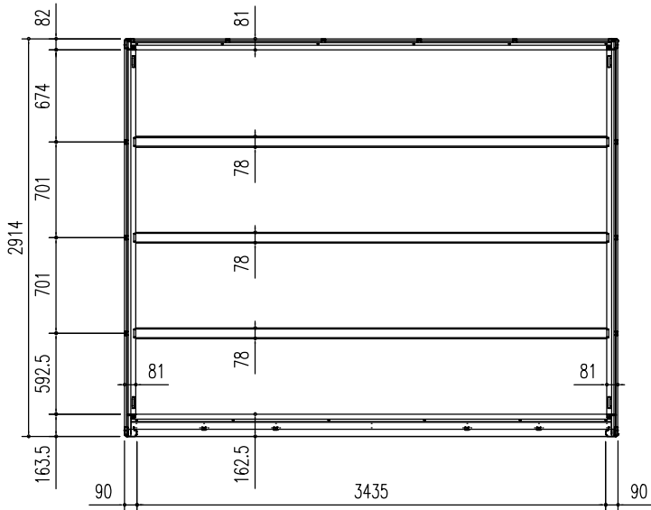
床 伏 図 (S = 1/50)
