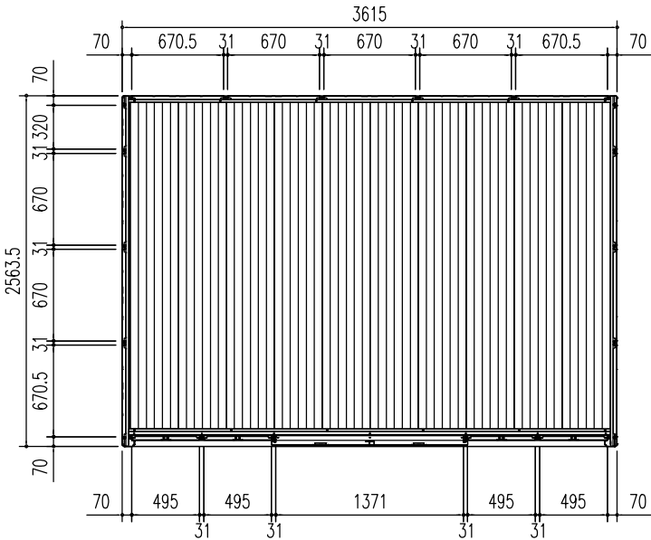
平 面 図 (S = 1/50)
