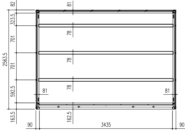
床 伏 図 (S = 1/50)
