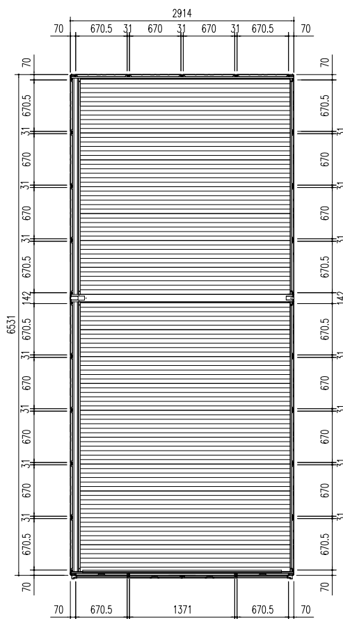
平面図 (S = 1/50)
