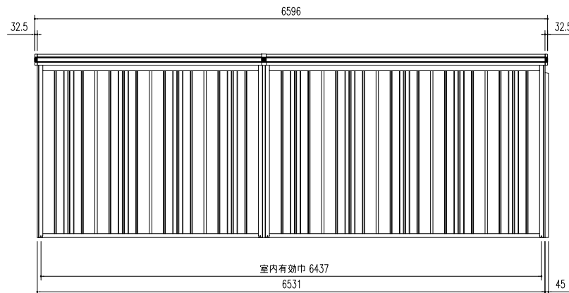
側面立面図 (S = 1/50)
