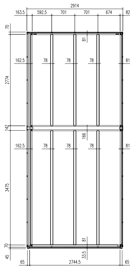
床伏図 (S = 1/50)
