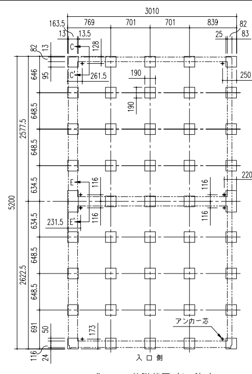
ブロック基礎伏図 (S=1/50) (内アンカー用)
