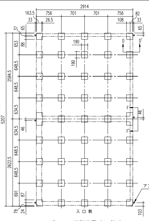
ブロック基礎伏図 (S=1/50) (外アンカー用)
