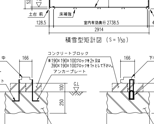
E ~ E' 断面 (内アンカー用)
