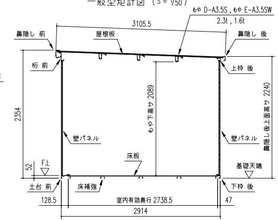
積雪型矩計図 (S=1/50)
