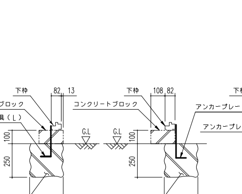
C ~ C' 断面 (内アンカー用)
