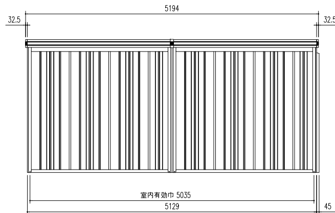
側面立面図 (S = 1/50)
