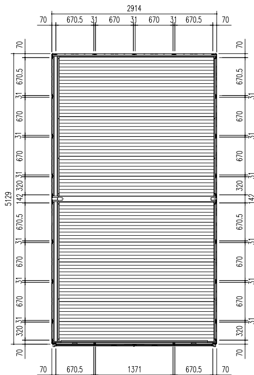
平面図 (S = 1/50)
