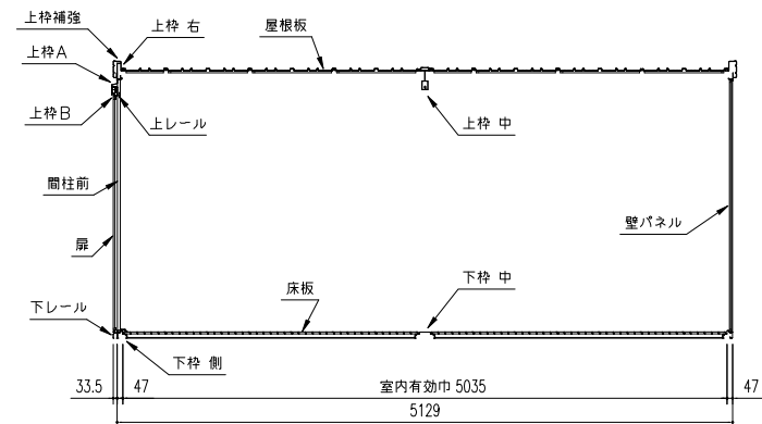
側面断面図 (S = 1/50)
