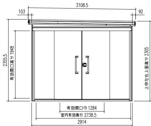
正面立面図 (S = 1/50)
