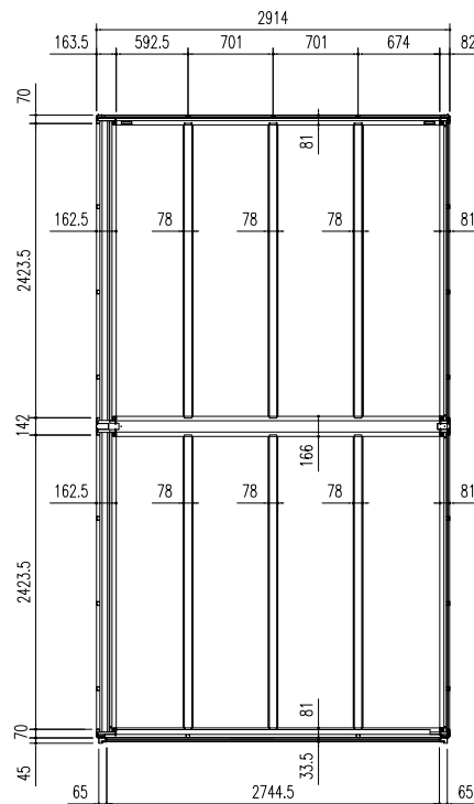
床伏図 (S = 1/50)
