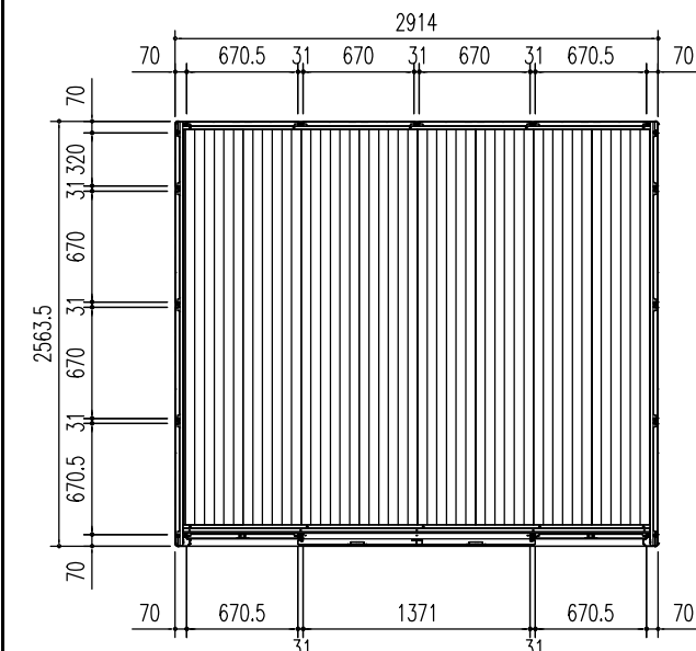
平面圖 (S = 1/50)
