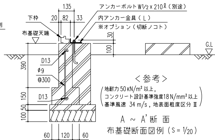
注1) 地耐力が50 kN/m 2 未満(30 kN/m 2 以上)の場合、底盤幅を300mmとし、かつ補助筋を入れて下さい。 注2) 寒冷地の場合、凍結深度等を考慮し、実情にあわせて設計して下さい。 注3) その他現地の実情にあわせて設計して下さい。
