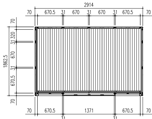
平面図 (S = 1/50)
