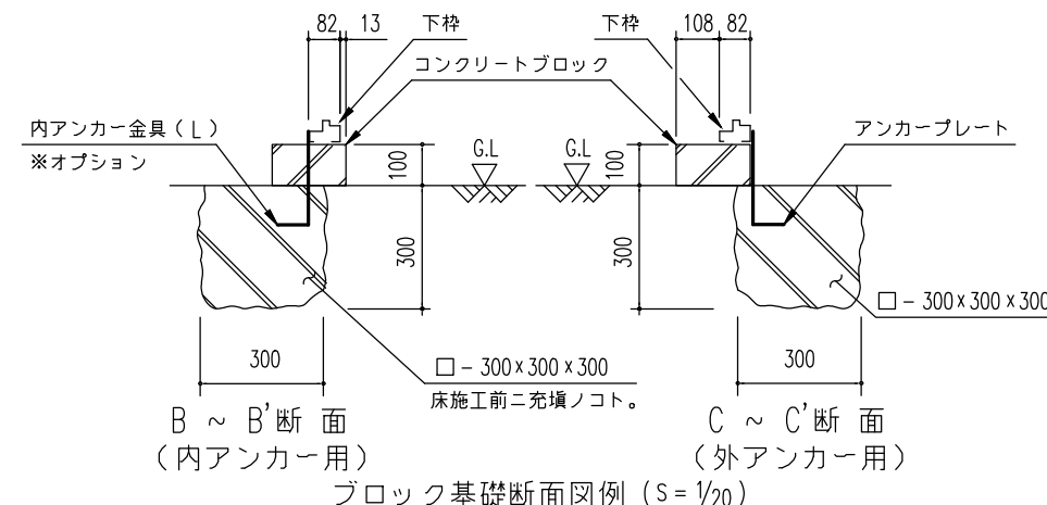
注1) 地耐力が50 kN/m 2 未満(30 kN/m 2 以上)の場合、底盤幅を300mmとし、かつ補助筋を入れて下さい。 注2) 寒冷地の場合、凍結深度等を考慮し、実情にあわせて設計して下さい。 注3) その他現地の実情にあわせて設計して下さい。
