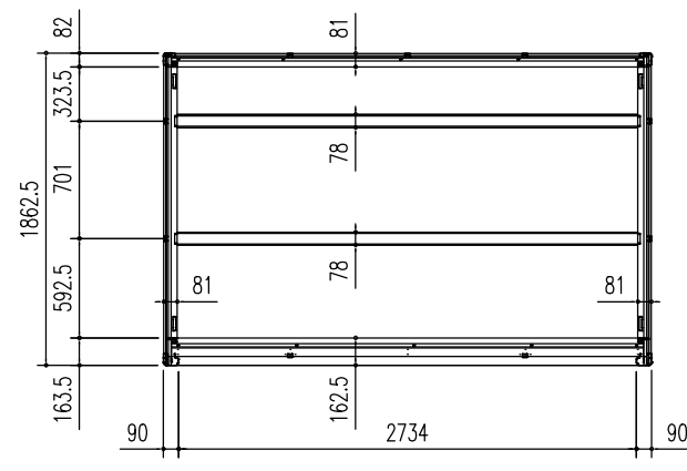
床伏図 (S = 1/50)
