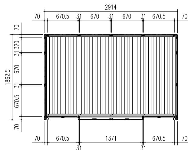
平面图 (S = 1/50)
