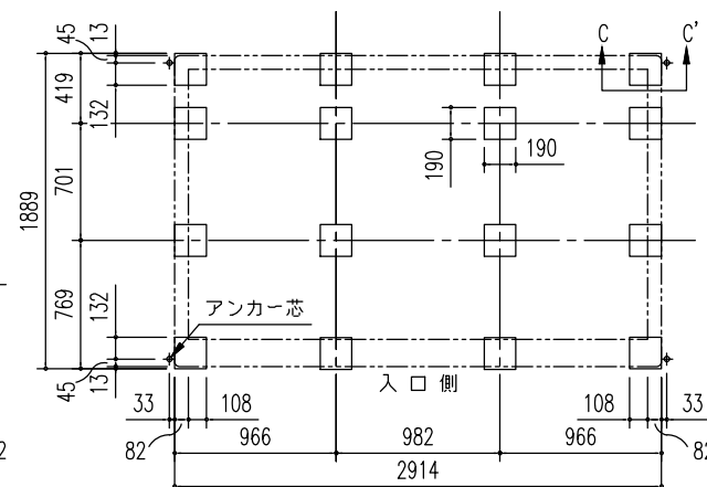
ブロック基礎伏図 (S = 1/50)
