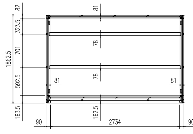
床 伏 図 (S = 1/50)
