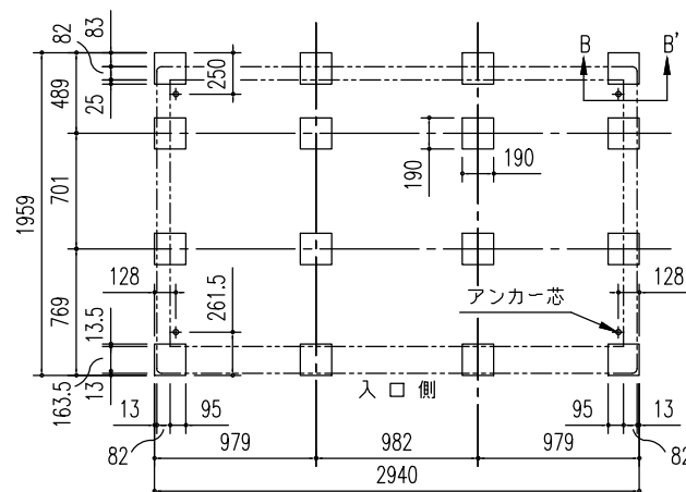
ブロック基礎伏図 (S = 1/50)
