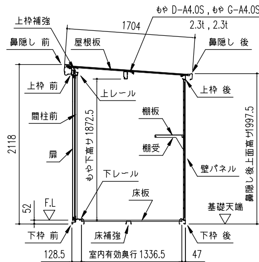
積雪型矩計図 (s = 1/50)
