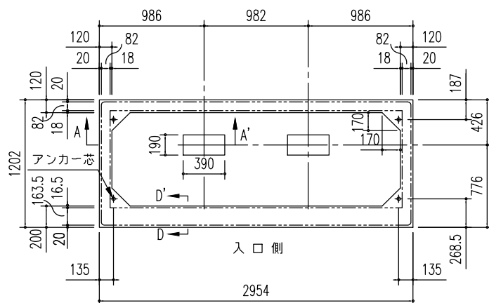
布基礎伏図 (S = 1/50) ※内アンカーセット(オプション) 別途必要
