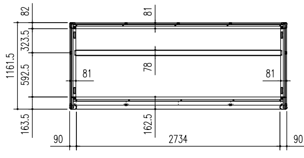
床伏図 (S = 1/50)
