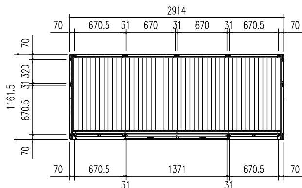
平面図 (S = 1/50)
