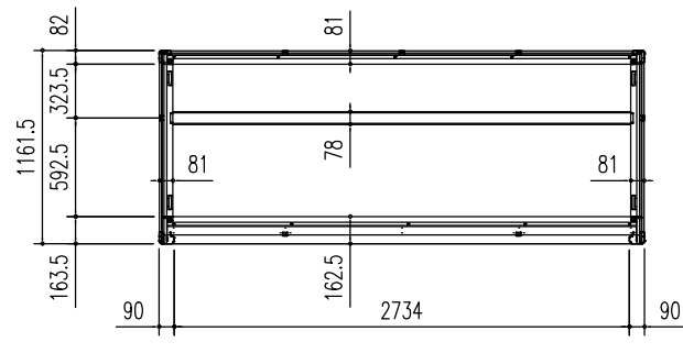
床伏図 (S = 1/50)
