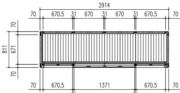
平面図 (S = 1/50)
