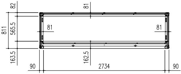
床 伏 図 (S = 1/50)
