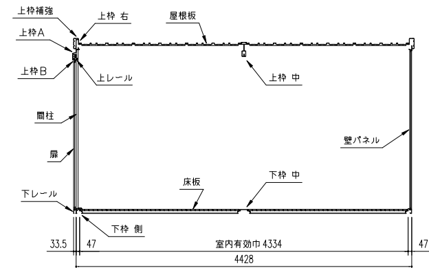
側面断面図 (S = 1/50)
