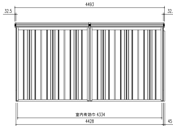
側面立面図 (S = 1/50)
