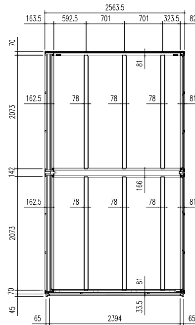
床伏図 (S = 1/50)
