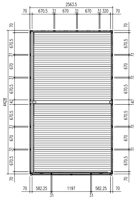
平面図 (S = 1/50)
