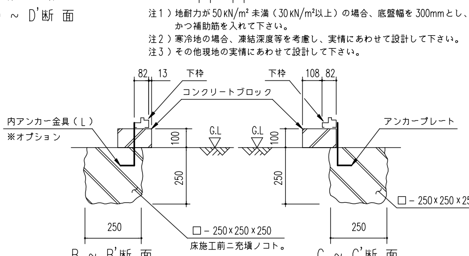
B ~ B' 断面 (内アンカー用)
