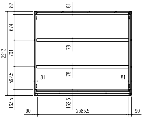
床伏図 (S = 1/50)
