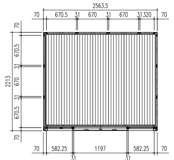
平面図 (S=1/50)
