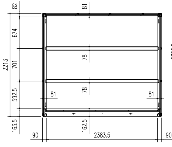
床伏図 (S=1/50)
