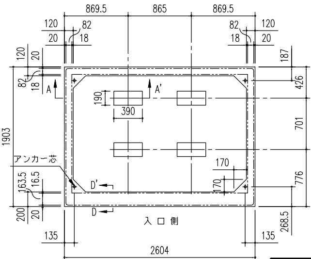
布 基 礎 伏 図 (S = 1/50)
