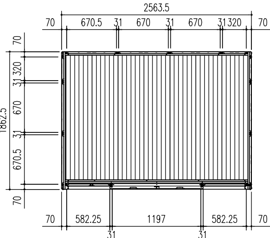
平面図 (S = 1/50)
