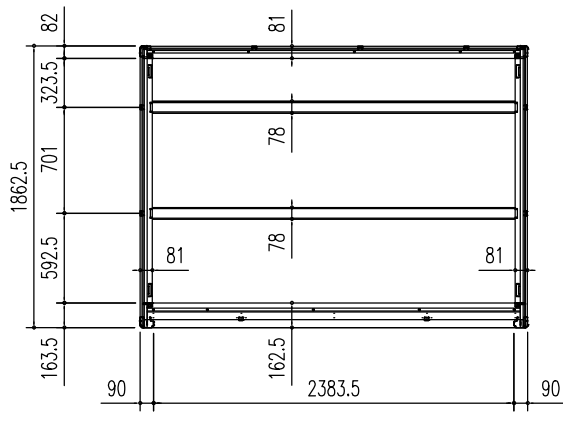
床 伏 図 (S = 1/50)
