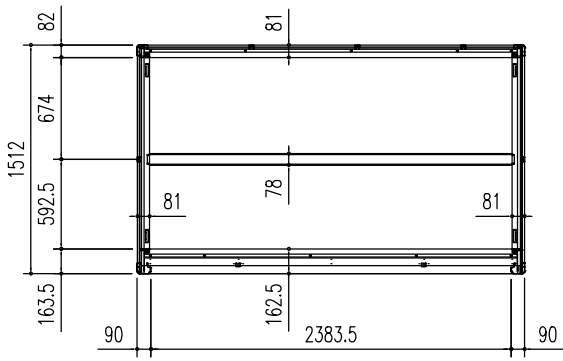
床 伏 図 (S = 1/50)
