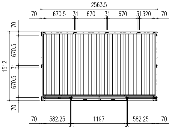
平面図 (S = 1/50)
