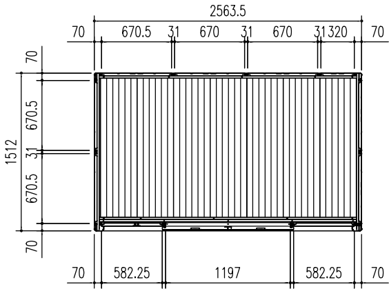
平面図 (S = 1/50)
