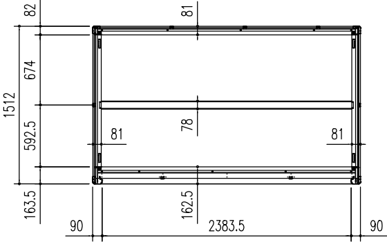
床伏図 (S = 1/50)
