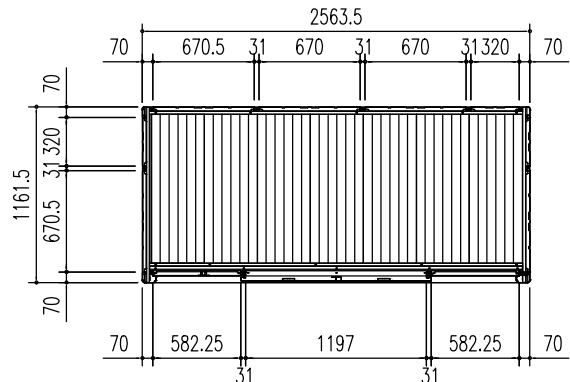
平面図 (S = 1/50)
