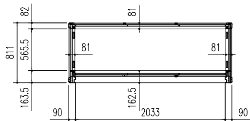
床 伏 図 (S=1/50)
